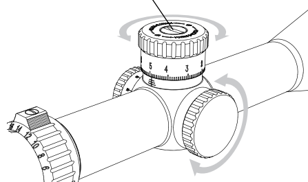
Vis de centre de la molette de hauteur
