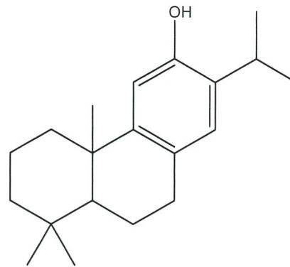
Ferruginol
