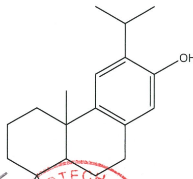
Ferruginol
