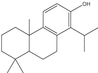
Totarol
