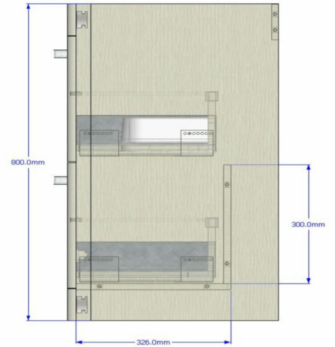
Right Elevation
