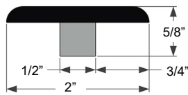
86" T-Mold
