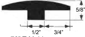
78" T-Mold
