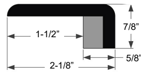
86" End Cap
