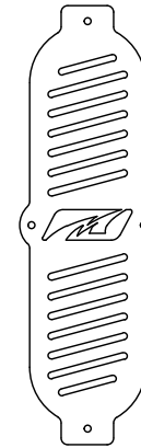
MB3044-03 Qty: 2
