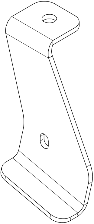
MB2146-01 Qty: 1
