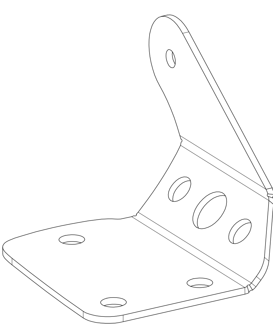
MB2017-01_MIR Qty: 1
