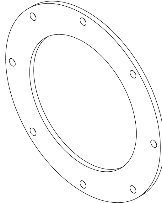
#MB5515-02 CLAMP RING QTY 1
