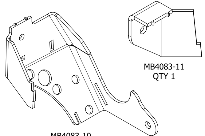
MB4083-10 QTY 1
