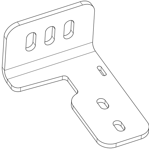
MB2412_MIR Qty 1
