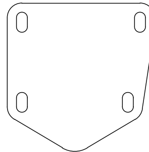
MB3019-01 Qty: 1
