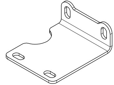
MB3018-01_MIR Qty: 1
