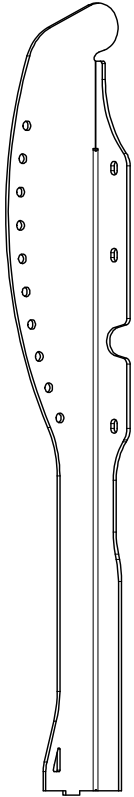
MB3006-01 Qty: 1
