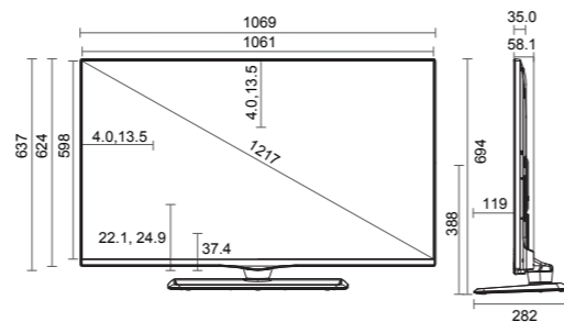
47F" 1069 x 694 x 282 / 18.3kg VESA(mm): 400 x 400
