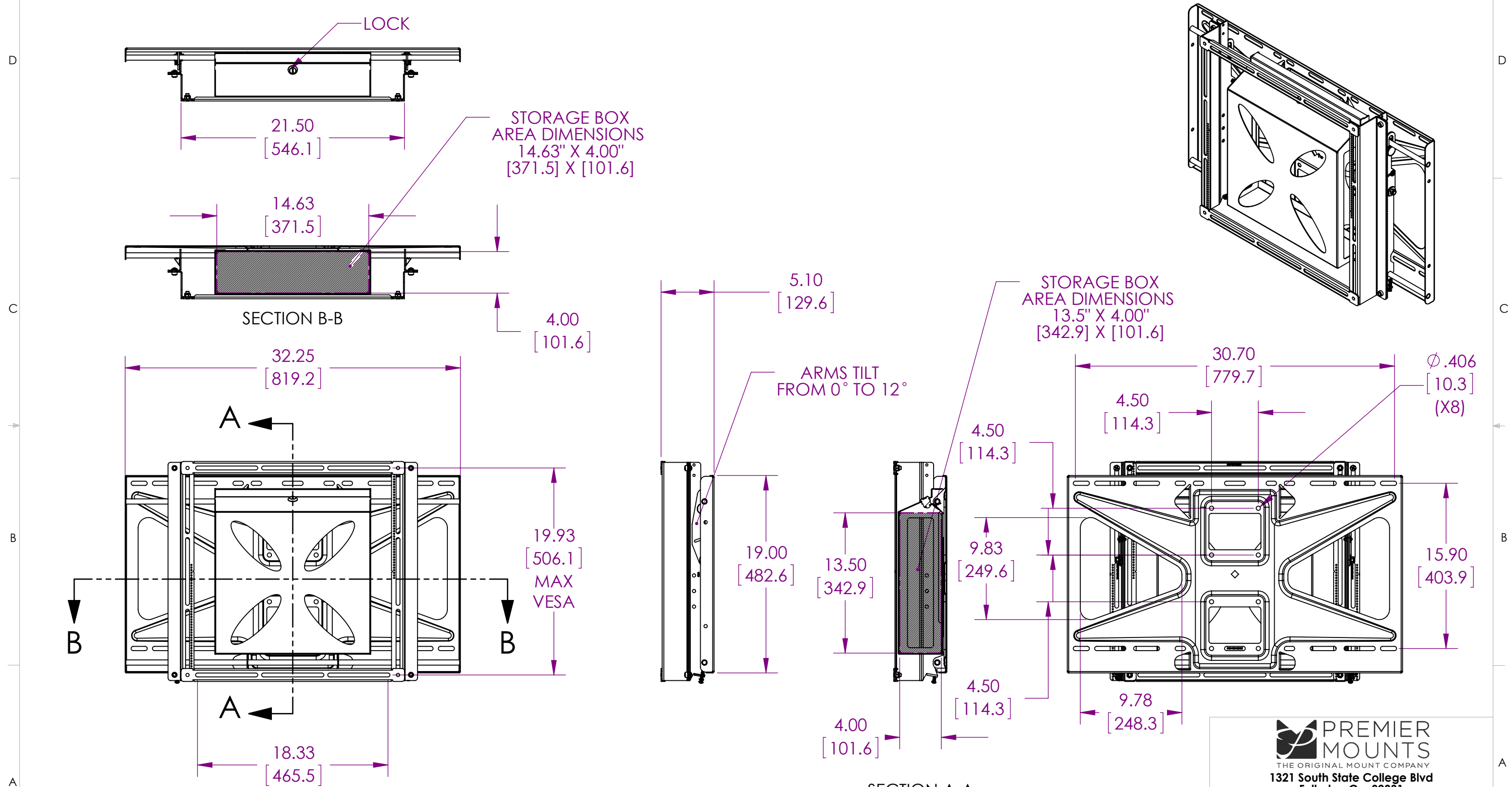
SECTION A-A
