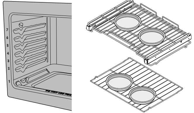
Figure 11: Position des casseroles pour de meilleurs résultats lors de la cuisson des gâteaux sur deux grilles.
