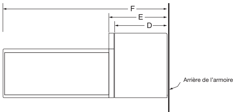
VUE LATÉRALE
