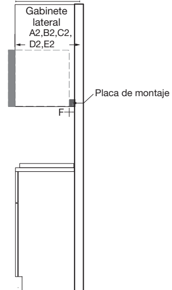
VISTA LATERAL
