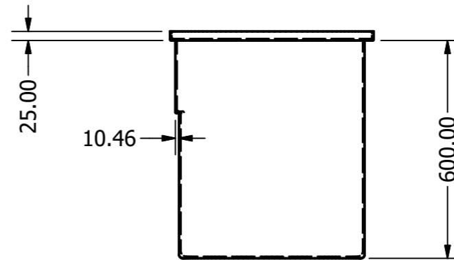
DETAIL A SCALE 0.14 : 1
