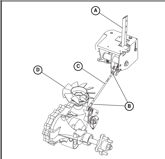
A. Steering control lever B. Jam nuts
