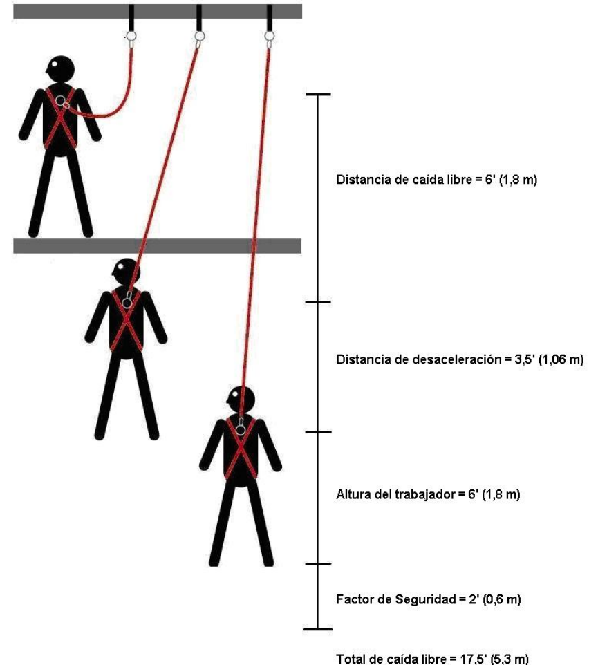
Figura 2.1: Diagrama de caída despejada
