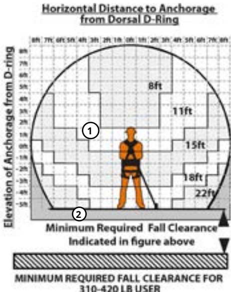
Figura 14 - Distancia despejada de caída mínima requerida de FT-X para usuarios de 310 a 420 libras (141 a 191 kg)
