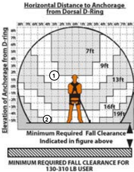
Figura 11 - Distancia despejada de caída mínima requerida de FT-X para usuarios de 130 a 310 libras (59 a 141 kg)
