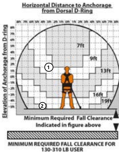
Figure 11 - Dégagement de chute minimum requis pour le FT-X pour les utilisateurs de 59 à 141 k (130 à 310 lb)
