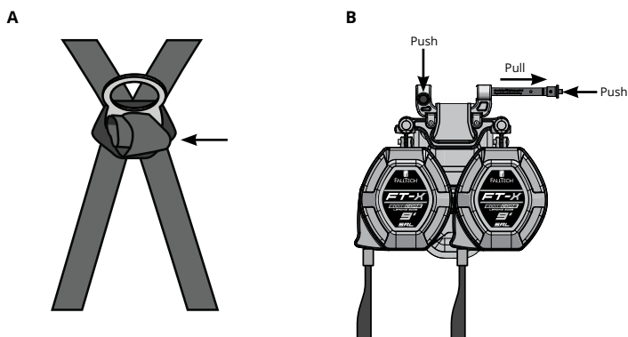
Figure 5 - Installation du bord d'attaque SRL-P de classe 2 FT-X Cable
