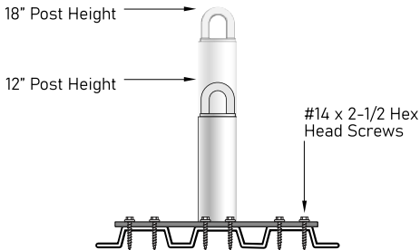
Single 20 ga. min. Deck Sheet
