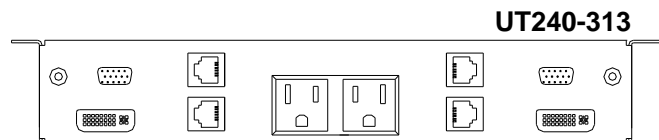
AC (2) DVI-I (2) Net (4) Audio (2) VGA (2)
