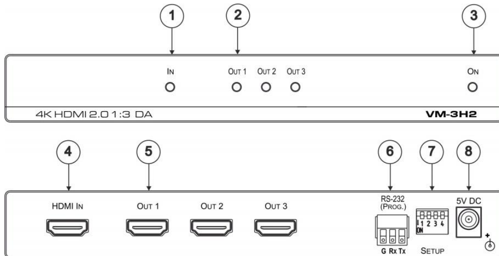
Figure 1: VM-3H2 4K HDMI 2.0 1:3 DA
