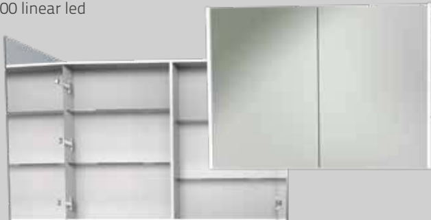
W990 x H700 x D145 mm
