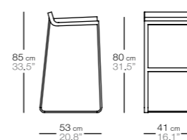
sit taburete con respaldo 78 back rest barstool 78
