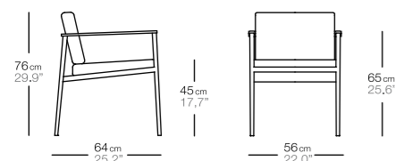
vint sillón armchair
