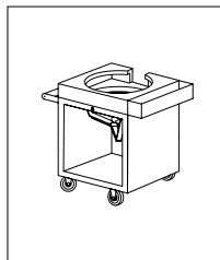
OFYR KAMADO TABLE CORTEN 65 PRO BOIS DE TECK KJ
