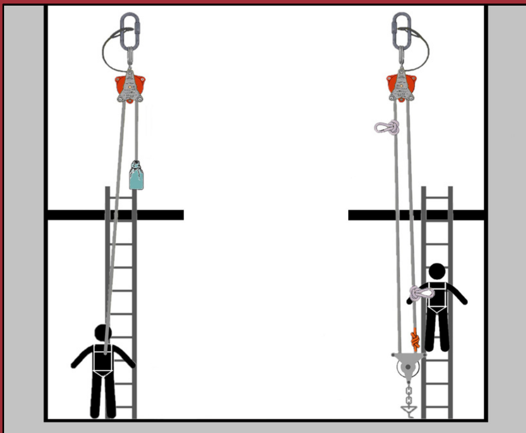
Gegengewichtsmontage
