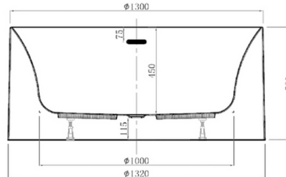
截面 F-F
