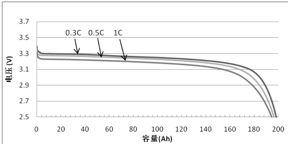
图 1. CA180F I 常温放电曲线
