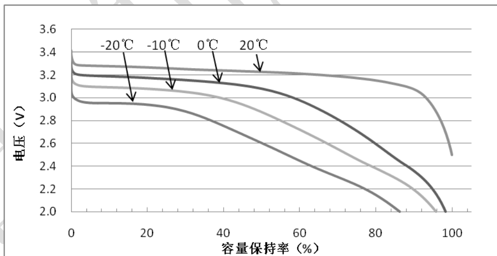
图 2. CA180F I 不同温度放电曲线
