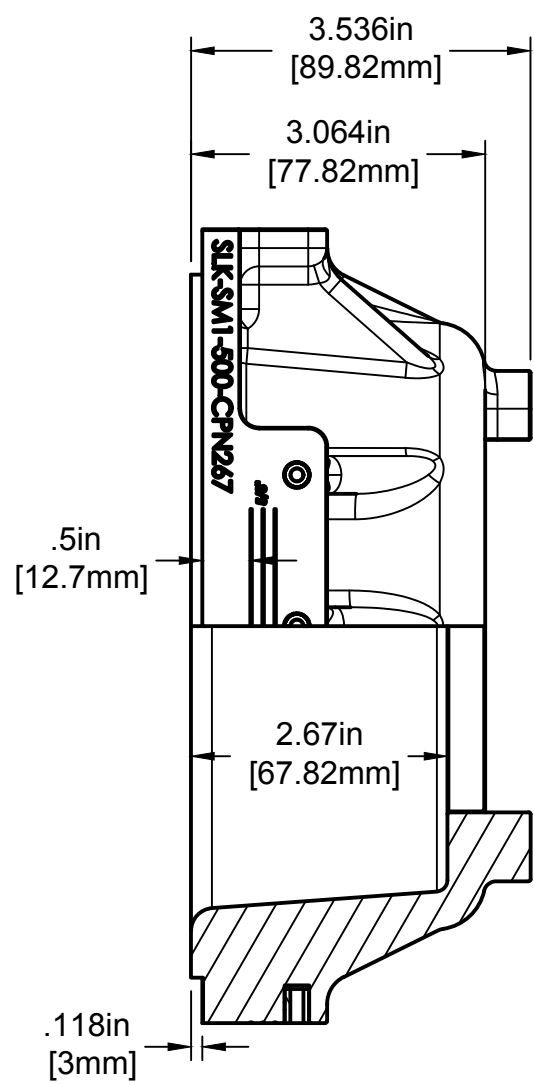
SECTION A-A SCALE 1:2
