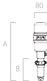
PIUSI 5.5:1 ST
