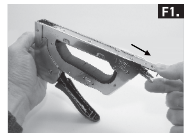
F1. Squeeze track release and pull out. Apriete la liberación de la pista y extráigala.
