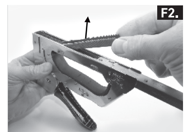
F2. Load staples with legs pointed up. Cargue grapas con las piernas hacia arriba.
