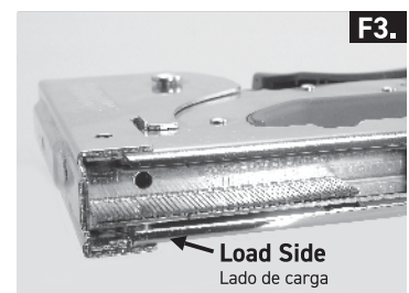
F3. Nails MUST contact the Load Side of chamber. Los clavos DEBEN entrar en contacto con el lado de la carga de la cámara.
