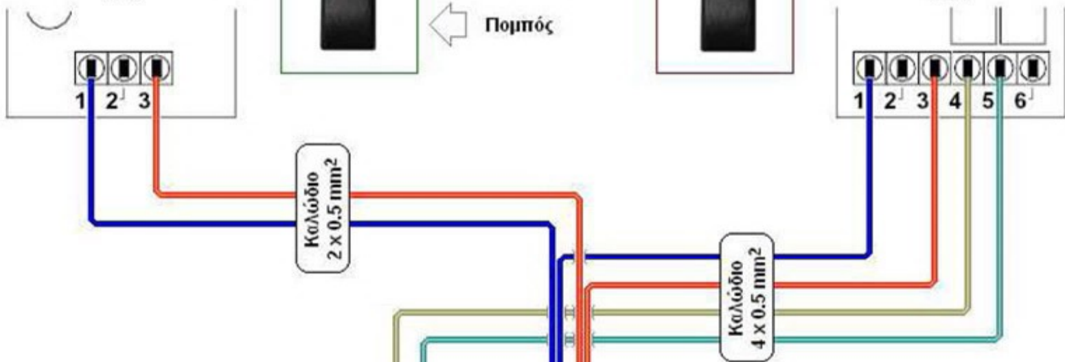
Πομπός φωτοκυτάρων ασφαλείας (TX)
