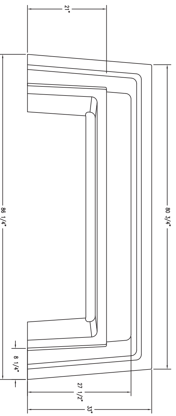
2 ELEVATION VIEW Scale: 1/8" = 1"
