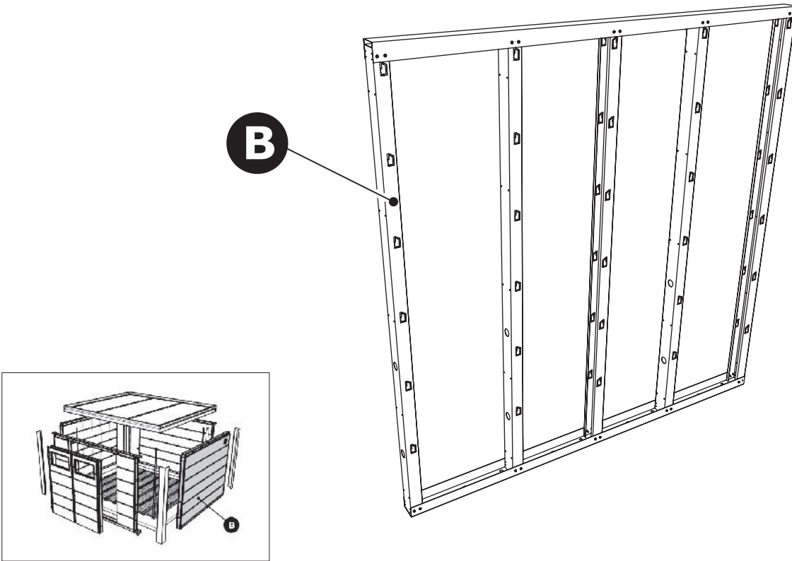
B Fachada / Fachada
