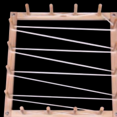
snovací rám Pro 11m osnovu.
