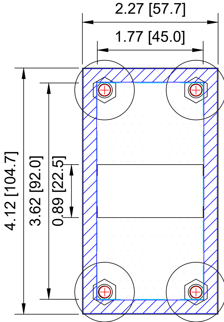
1/8 DIN Vertical to 1/32 DIN Horizontal Adapter Plate
