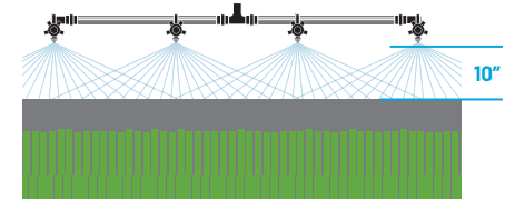
PATRÓN DE ASPERCIÓN EN 130° CON SUPERPOSICIÓN DEL 50% A MENOR ALTURA DEL BOTALÓN.
