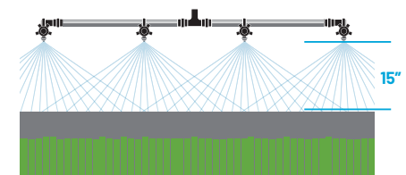
PATRÓN DE ASPERCIÓN EN 110° CON SUPERPOSICIÓN DEL 50% A MAYOR ALTURA DEL BOTALÓN.
