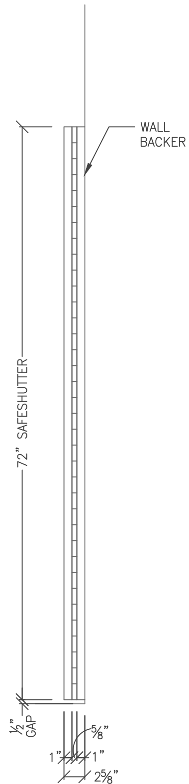
2 ELEVATION 2.5 SCALE: 1" = 1'-0"
