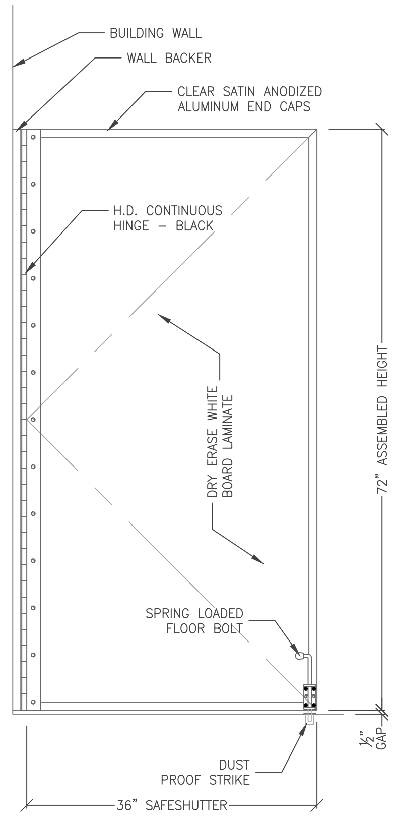
3 ELEVATION 2.1 SCALE: 1" = 1'-0"
