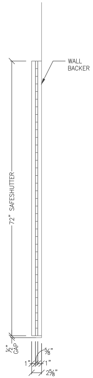
2 ELEVATION 2.1 SCALE: 1" = 1'-0"
