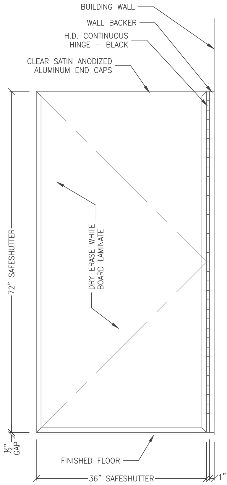
1 ELEVATION 2.1 SCALE: 1" = 1'-0"
