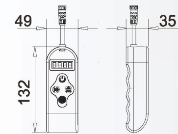
CTR-ADD-MR 单位/Unit : mm
