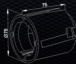
LWL-BF1/BF2 单位/Unit: mm 预埋件 / Embedded Part
