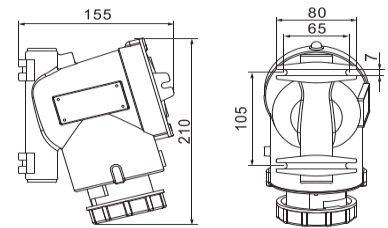
Socket
