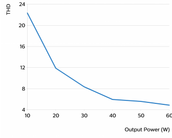
THD 与输出功率
