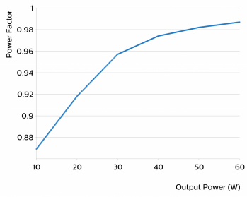
功率因数与输出功率
