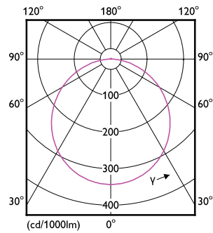
Downlight DN020 G3 CW 18W D175 SNI
