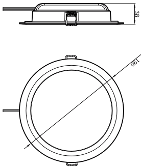
DN020B G3 LED15/CW 18W 220-240V D175 SNI
