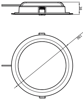
DN020B G3 LED15/WW 18W 220-240V D175 SNI
