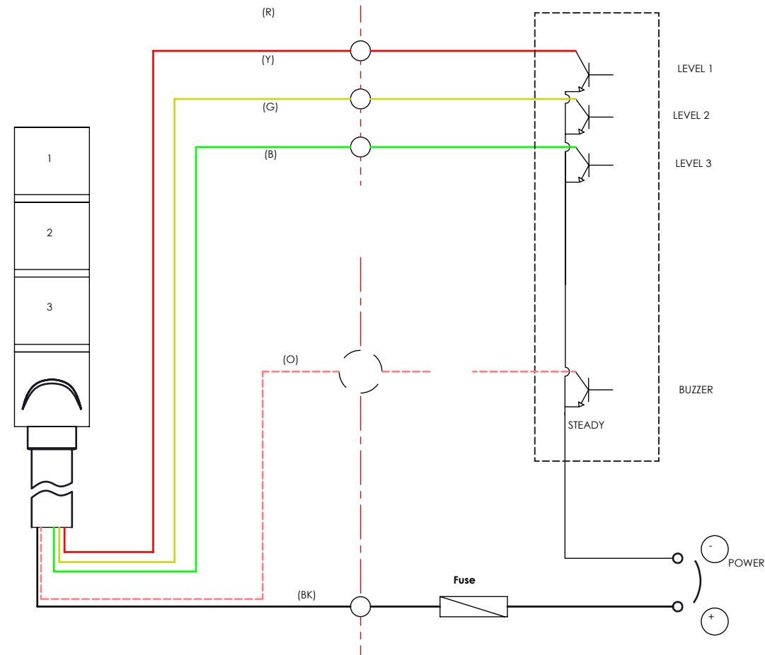
NPN
