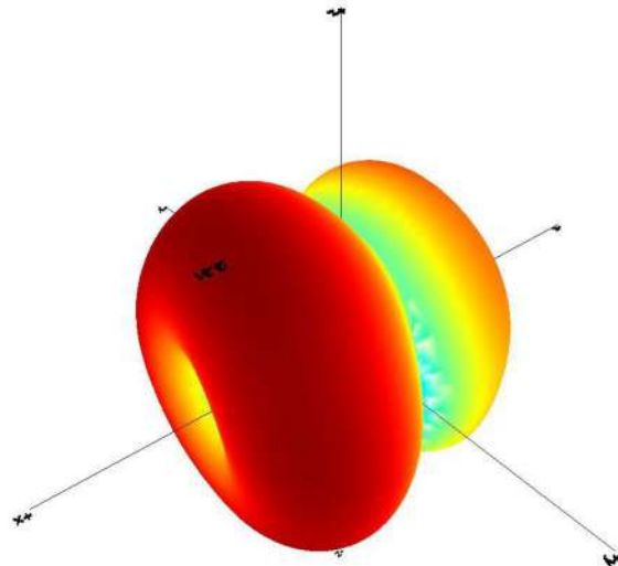
2170MHz
