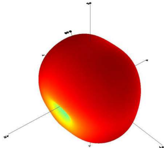
960MHz
