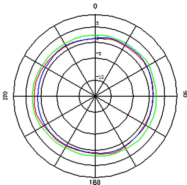
水平面方向图(2.4G天线) Horizontal Pattern
