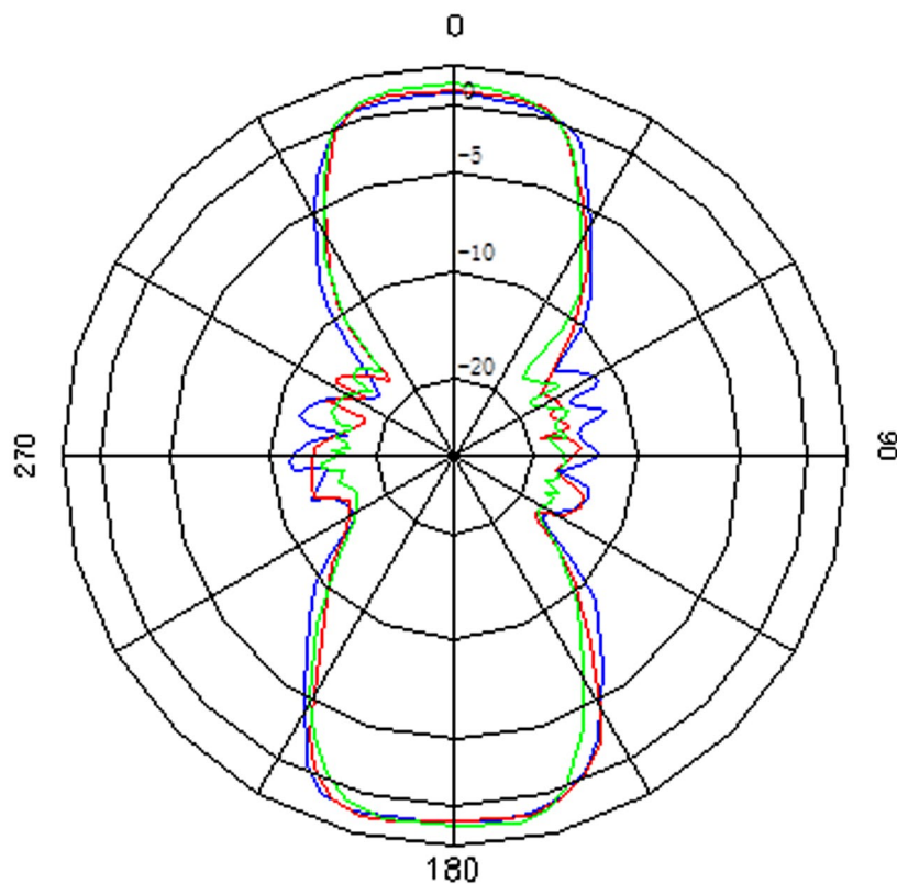
垂直面方向图 Vertical Pattern
