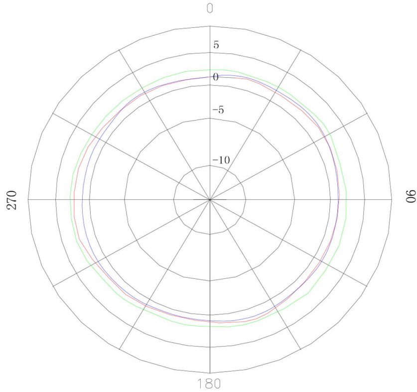
水平面方向图 (2.4G天线) Horizontal Pattern
