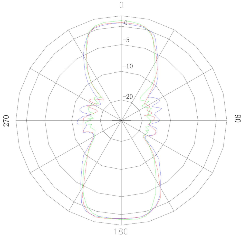
垂直面方向图 Vertical Pattern
