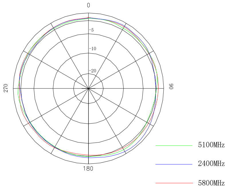
垂直面方向图 Vertical Pattern
